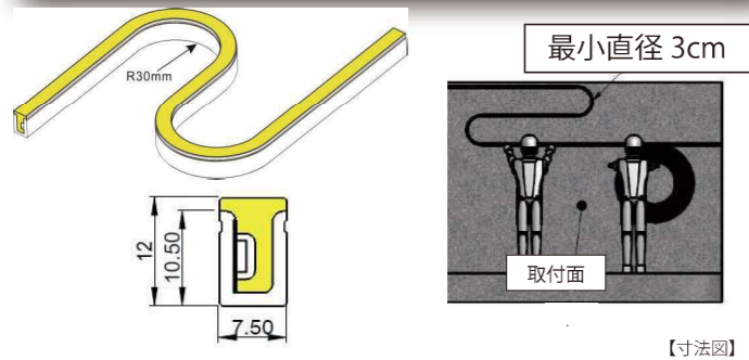
【寸法図】
