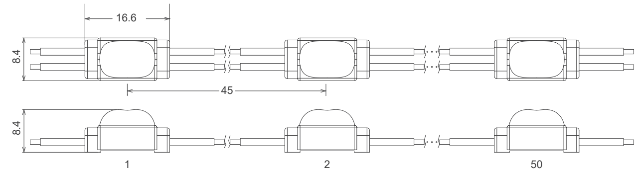
製品寸法図 (mm)
