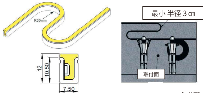
【寸法図】
